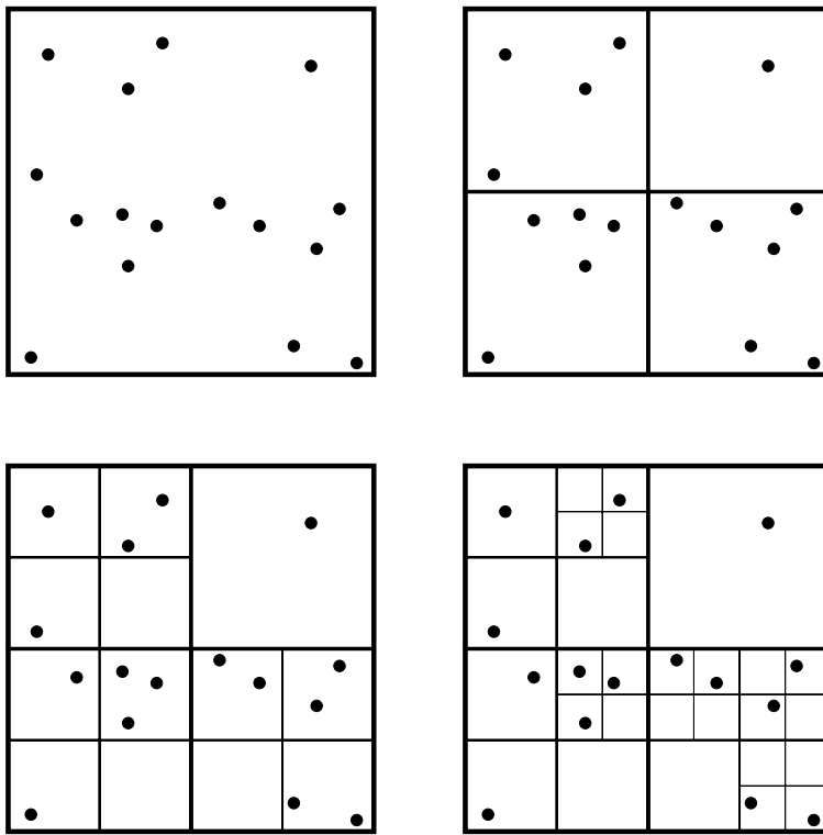
図 4.6: ツリー構造の構築
