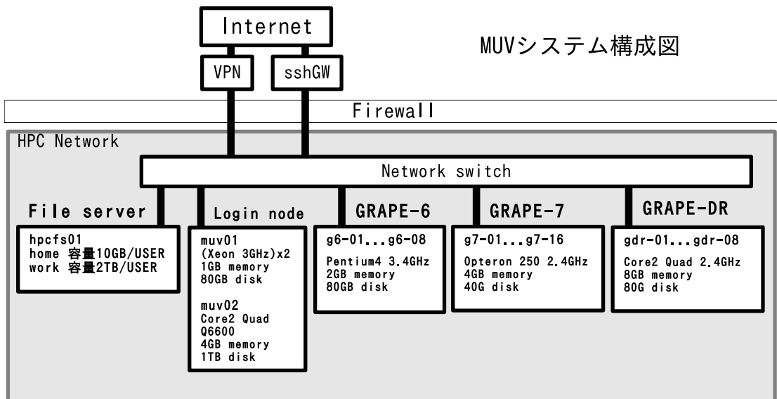
図 4.4: 国立天文台 GRAPE システム ネットワーク構成
