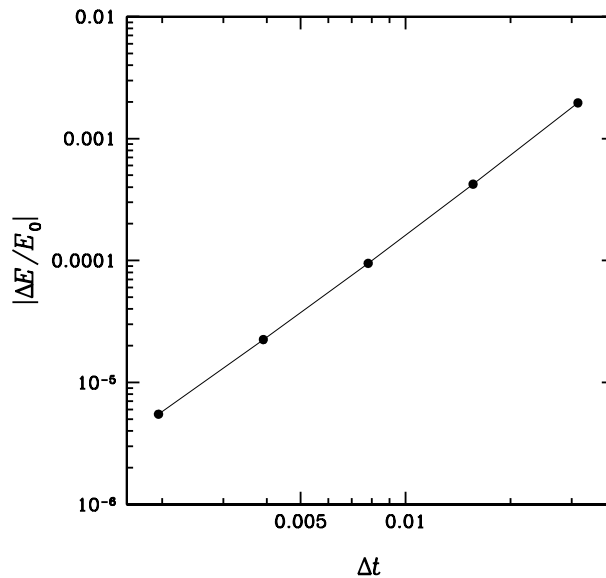
図 5.4: エネルギーの相対誤差のタイムステップへの依存
