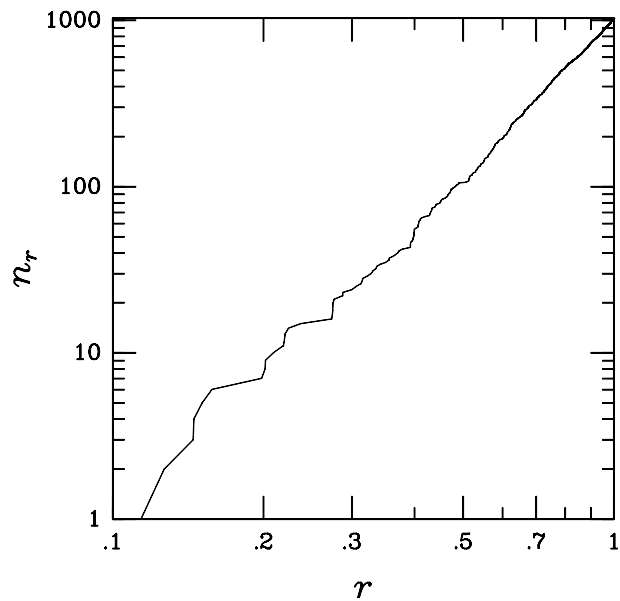
図 5.3: 粒子数 1024 の場合の一様球の r - n_r 図
