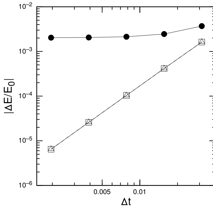
図 5.4: エネルギーの相対誤差のタイムステップへの依存 ( \Delta はホストコンピュータのCPUのみ、 \square はGRAPE ライブラリからGPUを使用、 \bullet はGRAPE-9を使用)
