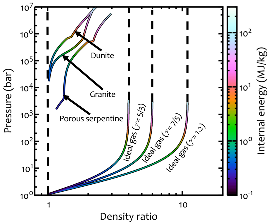
図 3.1.1. 種々の物質の規格化密度-圧力平面における Hugoniot 曲線. 1 bar = 10^5 Pa.
