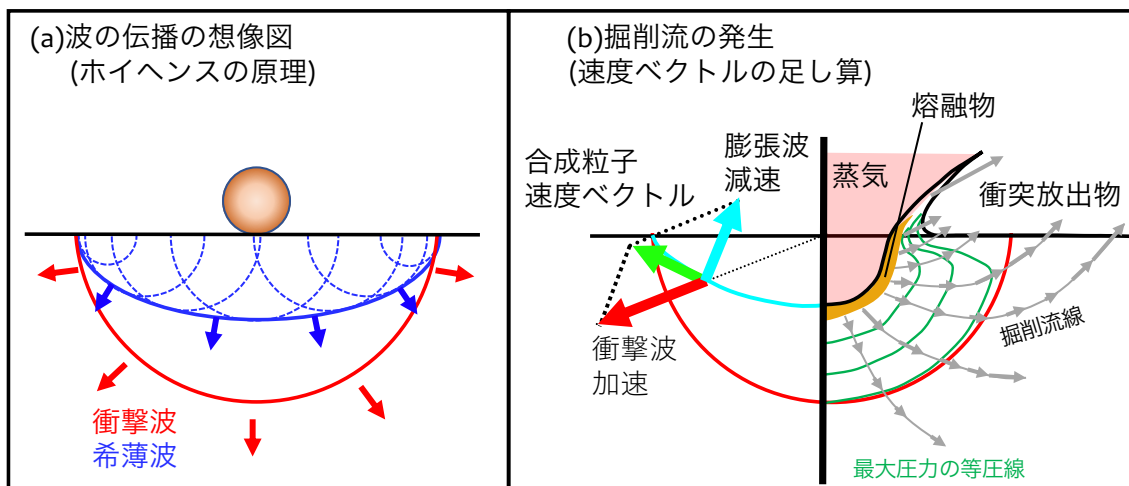
図 3.1.2. (a)衝撃波を追いかける希薄波発生の模式図。青点線は自由表面から発生したホイヘンスの素元波。 (b) 衝撃波加速と膨張波減速による粒子速度変化の模式図。クレータの科学, 図 3.1 と 3.4, [水谷, 1980]と Impact cratering, Fig.5.9 [Melosh, 1989]を参考にした。
