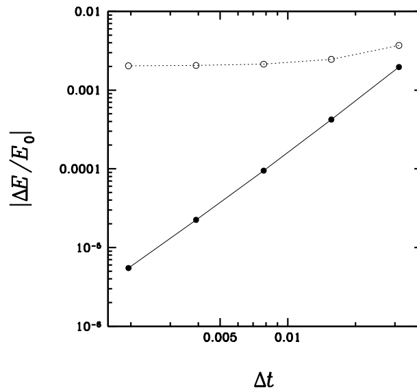
図 5.4: エネルギーの相対誤差のタイムステップへの依存 (●はホストコンピュータのみ、○は GRAPE-9 を使用)
