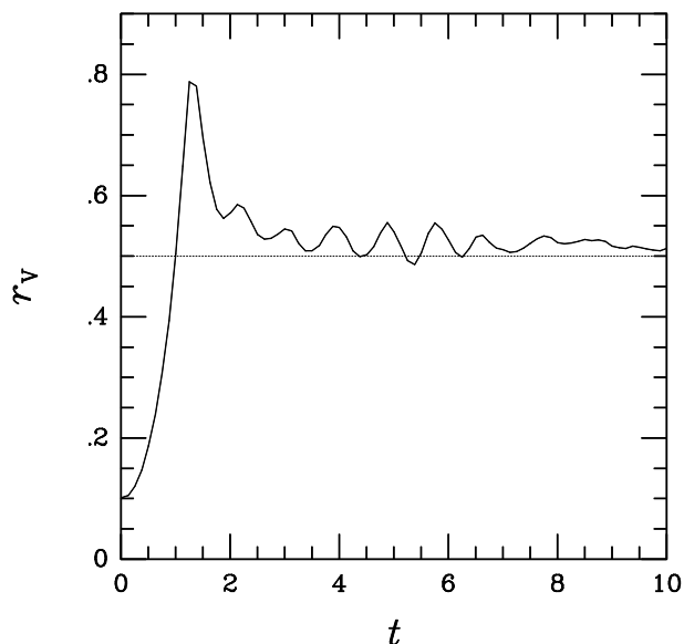
図 5.5: ビリアル比の時間進化
