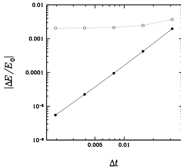
図 5.4: エネルギーの相対誤差のタイムステップへの依存 ( はホストコンピュータのみ、 は GRAPE-9 を使用)
