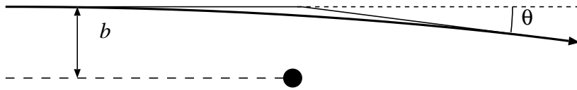
図 2.1: 2 体散乱
